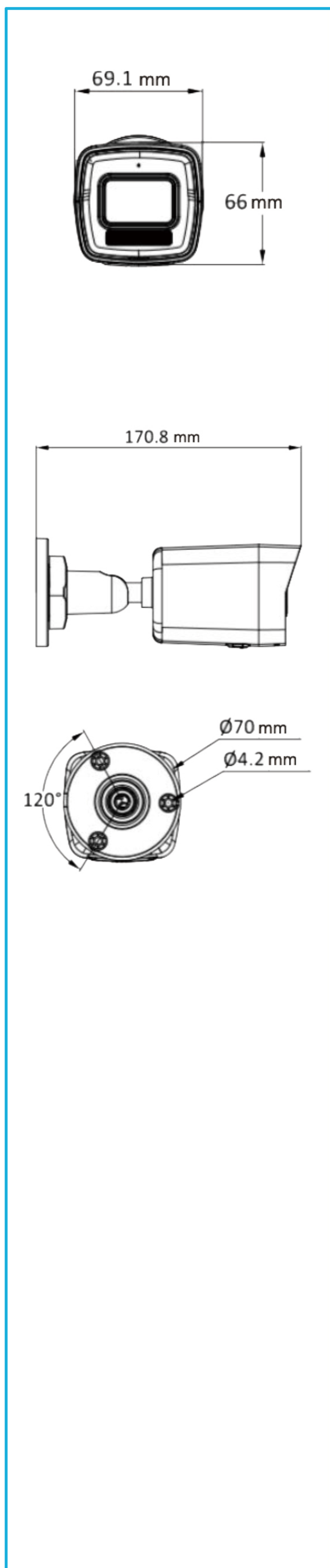
尺寸示意圖
